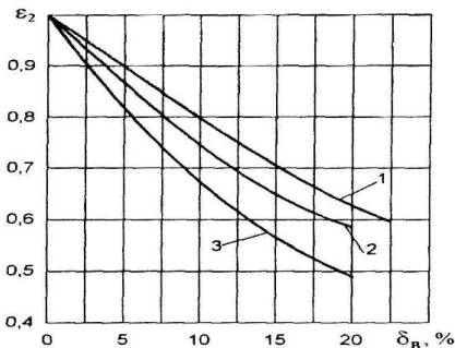
Рис. 6. График определения значений коэффициента \varepsilon_2 : 1 – газ, 2 – мазут, 3 – газ, \sigma_{в.} – доля воздуха, подаваемого помимо основных горелок
